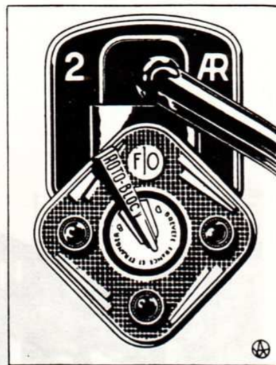
Le Rotobloc pour Citroën traction avant bloque le levier des vitesses en marche arrière.
